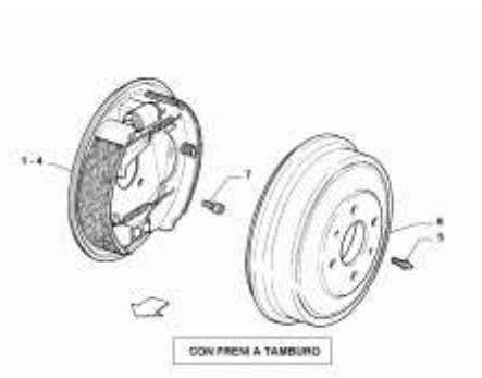
33125/00 - REAR WHEEL BRAKES (Var.1/Rev.0)
